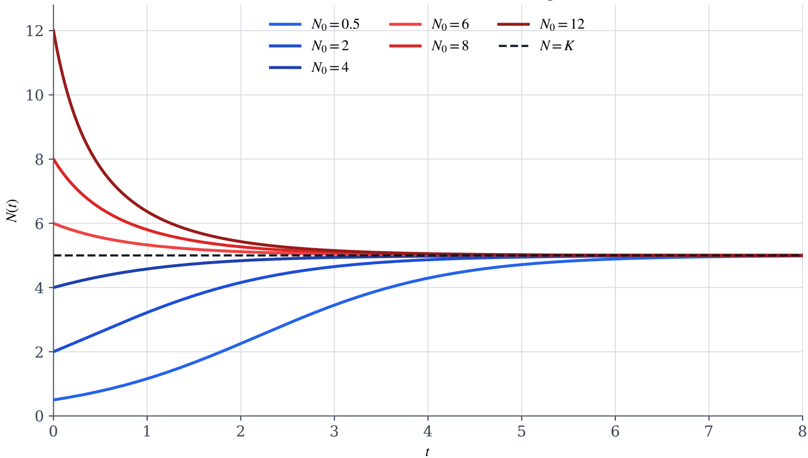
Familia de soluciones del modelo logístico
